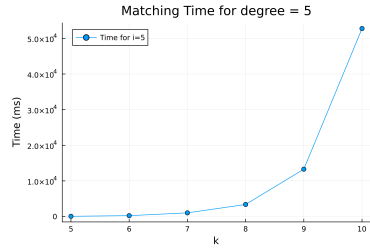
(e) Czasy dla i = 5
