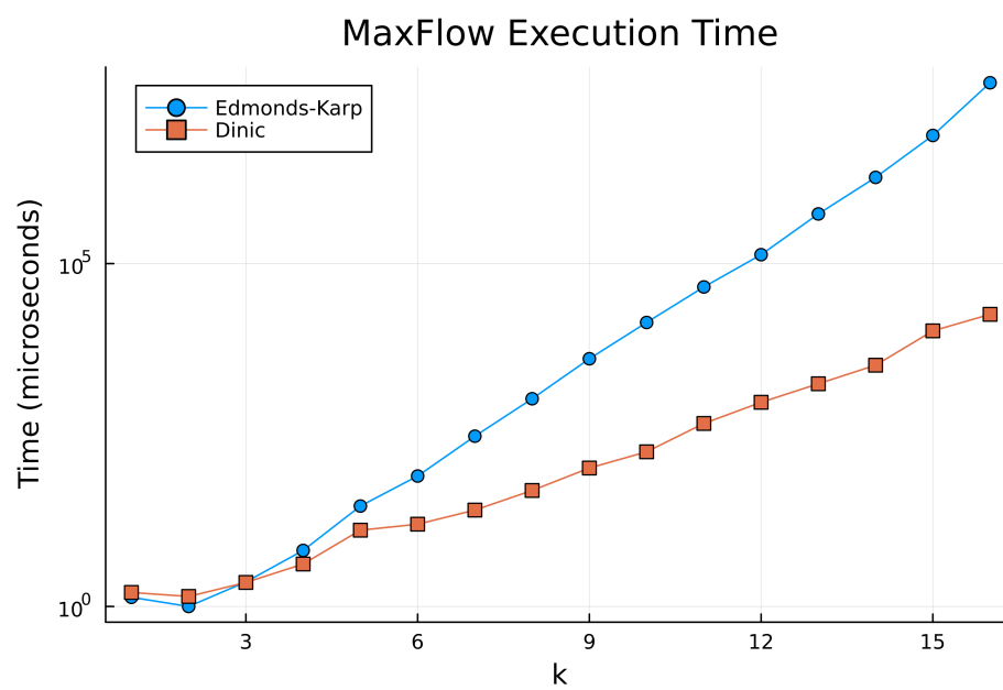
Rysunek 1: Wykres czasu względem k
