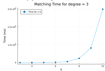
(c) Czasy dla i = 3
