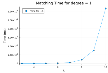
(a) Czasy dla i = 1
