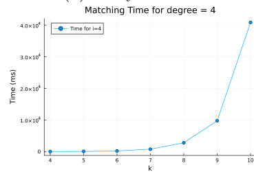
(d) Czasy dla i = 4
